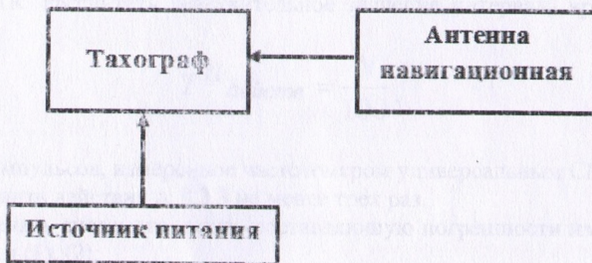
Рисунок 1 – Схема проведения измерений при проверке работоспособности
